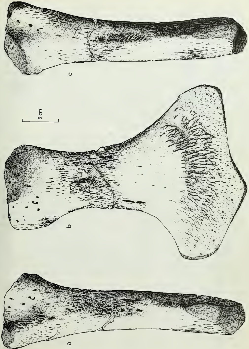
Fig. 15 Cryptoclidus eurymerus (Phillips), H.M.G. V. 1104. Left humerus: a, posterior; b, ventral; c, anterior aspect.
