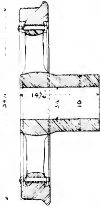
Fig. 436. MANHATTAN WHEEL.
